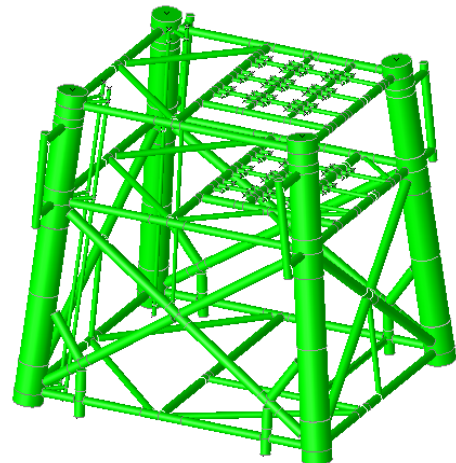
BZ28-2S WHPB导管架模型
