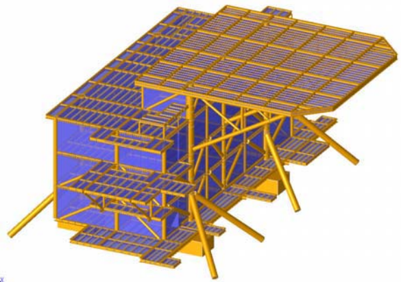
LQ MODEL 拖航模型
