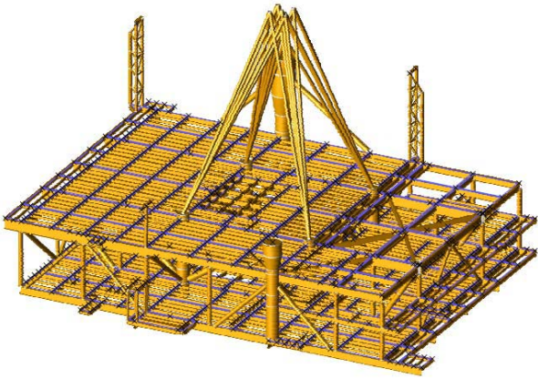
UPPER MODEL 吊装模型
