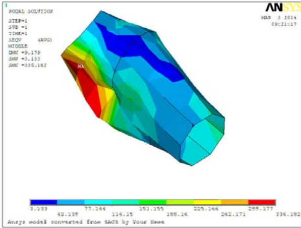
ANSYS 模型分析
