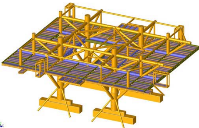
MSF MODEL 拖航模型
