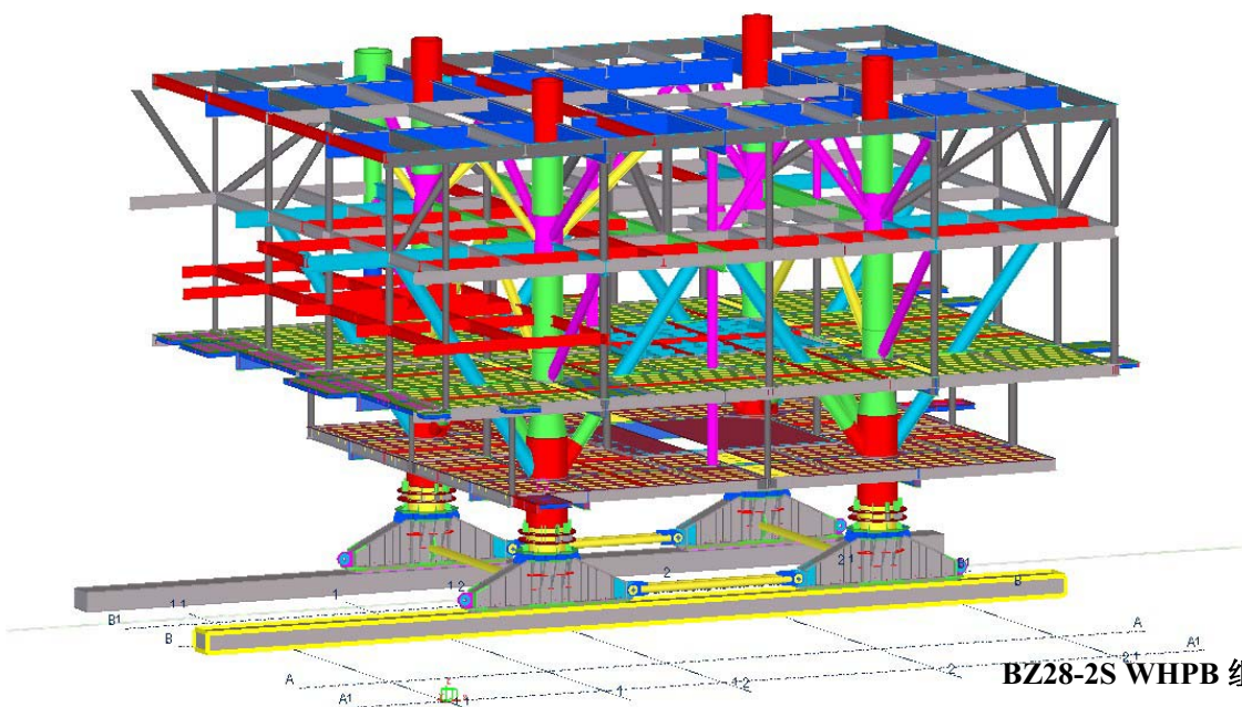
渤中28-2S WHPB--3#片建造
