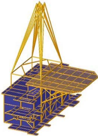
LQ MODEL 吊装模型
