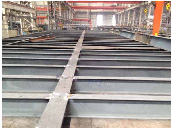
渤中28-2S WHPB--5#片建造
