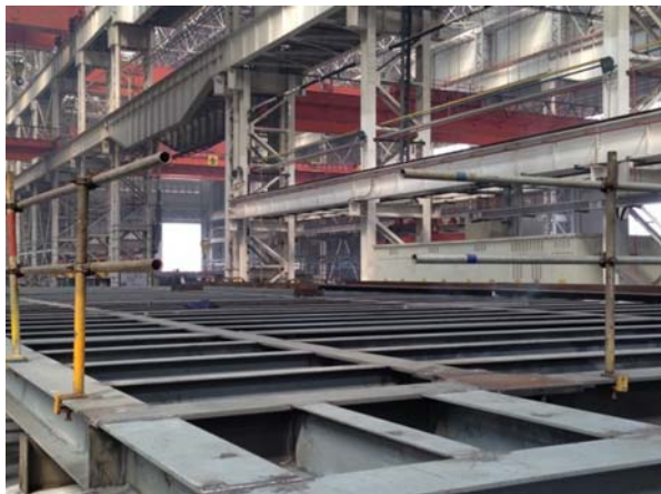
渤中28-2S WHPB--3#片建造
