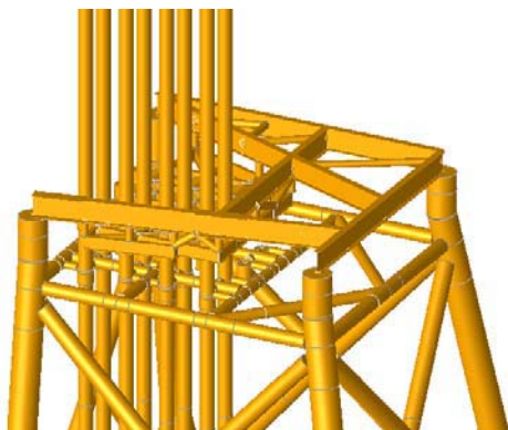
SACS 模型分析
