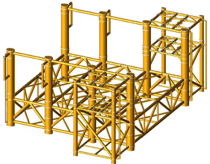
BZ34-2/4 CEPA导管架模型
