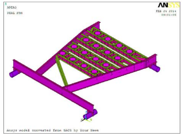
ANSYS 模型分析
