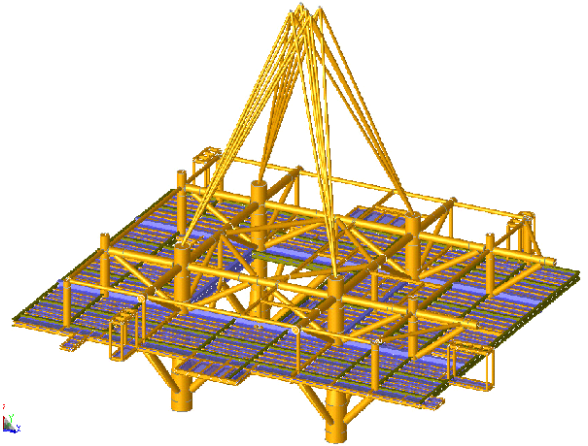
MSF MODEL 吊装模型
