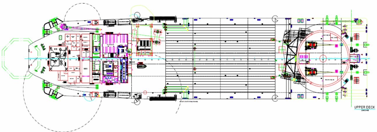
蓝琼系泊项目船图
