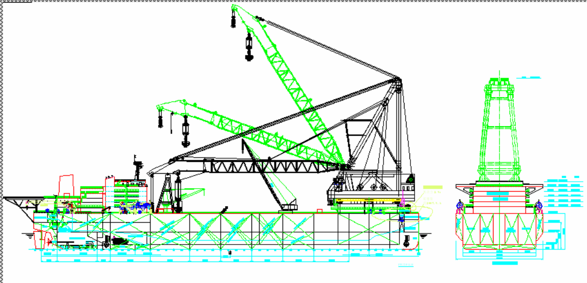
蓝琼系泊项目船图
