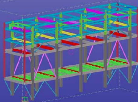
SZ36-1 WHPK XSTEEL模型
