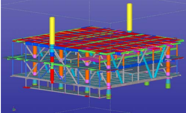
JZ25-1S CEP XSTEEL模型
