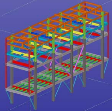
PIPERACKS XSTEEL 4C模型
