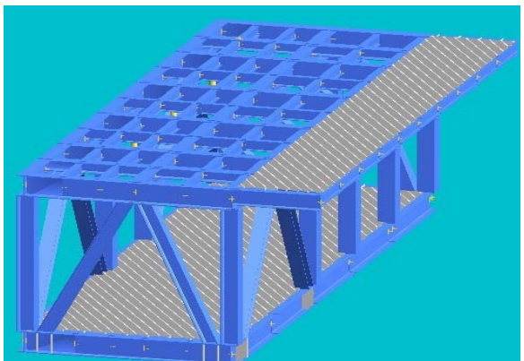
化学剂注入撬块 PDMS模型
