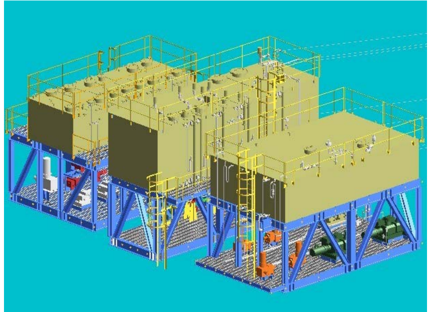
化学剂注入撬块 PDMS模型
