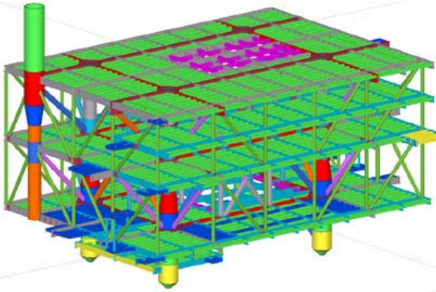
JX1-1 WHPB XSTEEL模型
